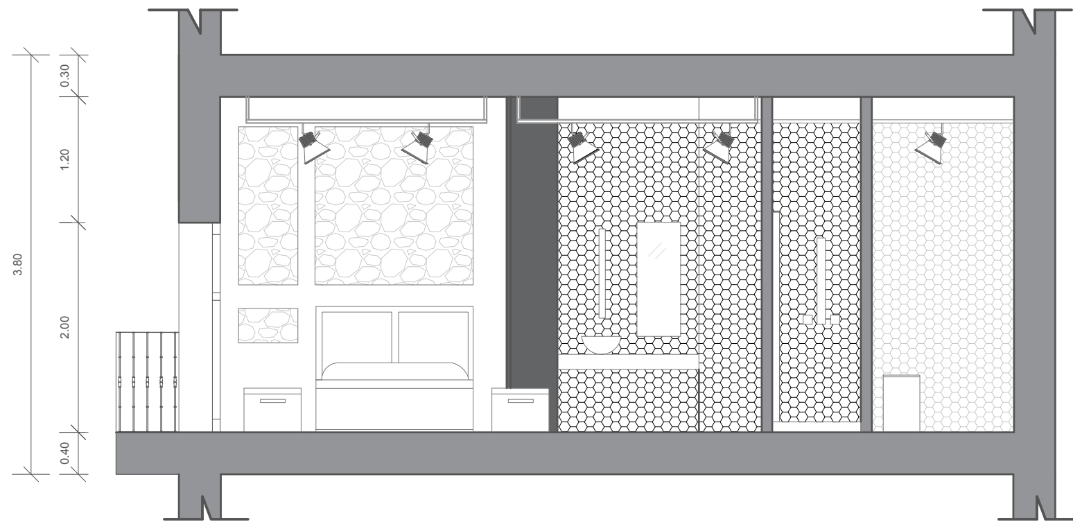
Sección CC'' E:1/50
