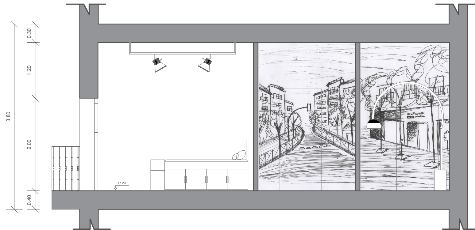
Sección DD'' E:1/50
