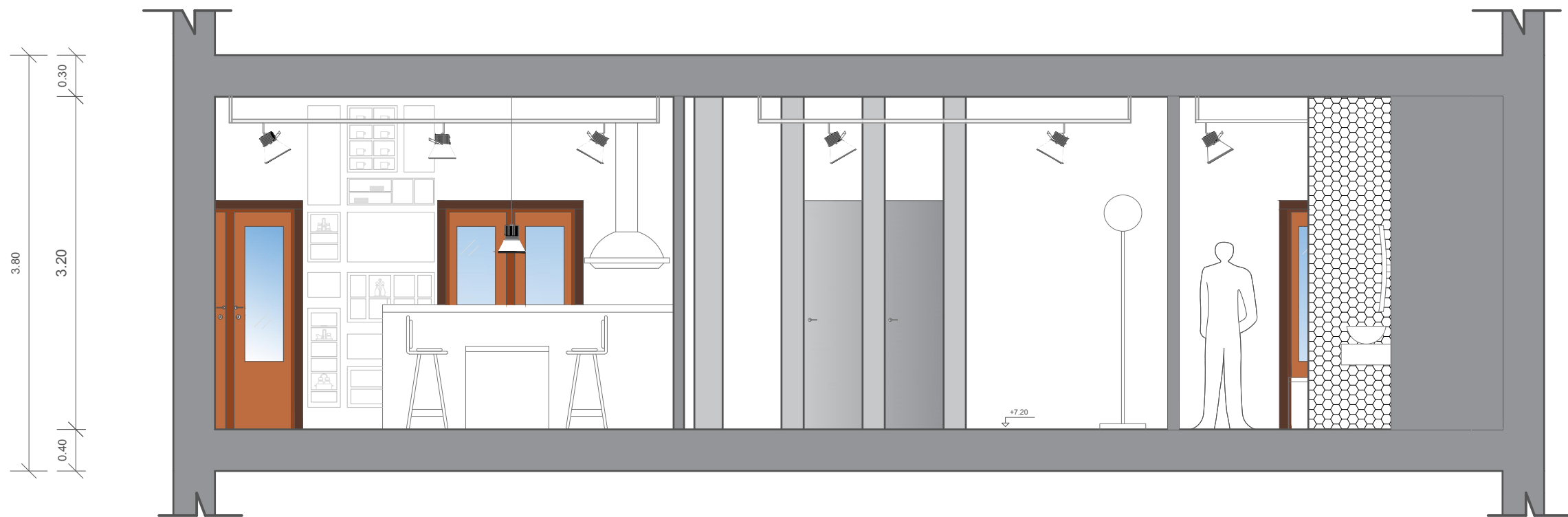
Sección AA'' E:1/50
