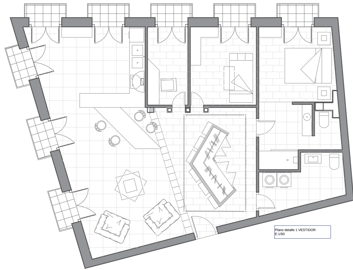
Planta de Distribución Renov. Vivienda C/Fuencarral nº122 E:1/100
