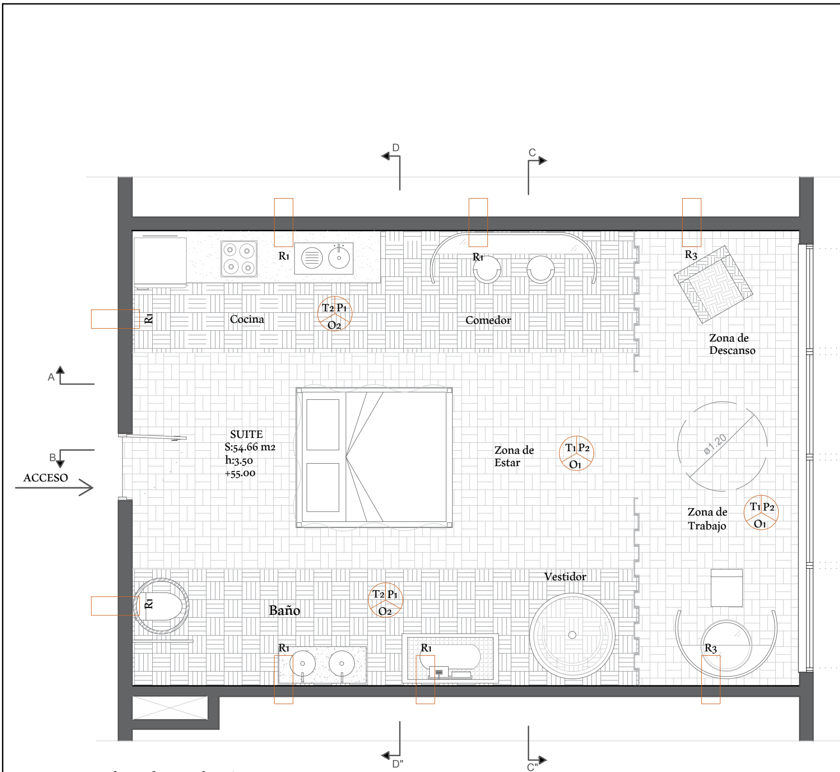
Planta de Distribución Escala: 1/50
