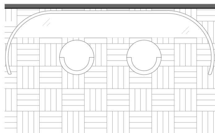
Detalle mobiliario-Zona Comedor E:1/25
