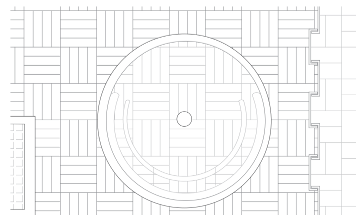
Detalle mobiliario-Zona Vestidor E:1/25
